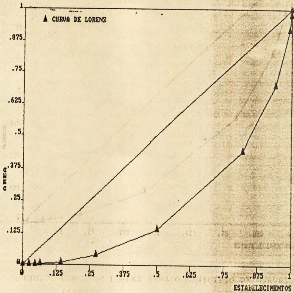
FIG.6: CURVA DE LORENZ PARA O MUNICÍPIO DE GURUPI (1975).
