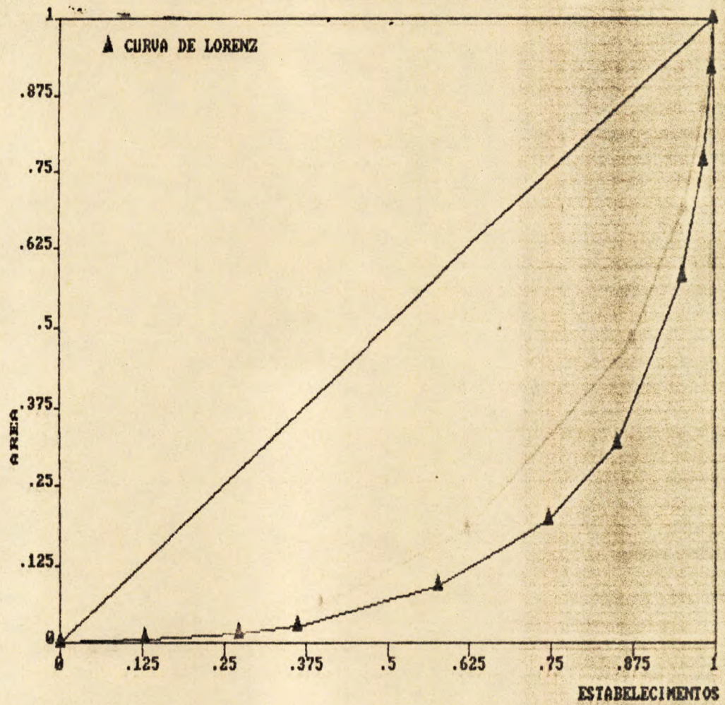
FIG.4: CURVA DE LORENZ PARA O MUNICÍPIO DE GURUPI (1960).
