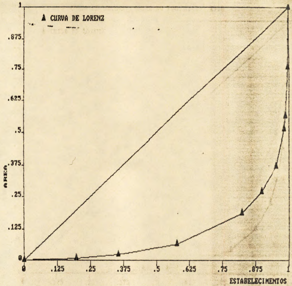
FIG.2: CURVA DE LORENZ PARA O MUNICÍPIO DE AXIXÁ DO TOCANTINS (1975).
