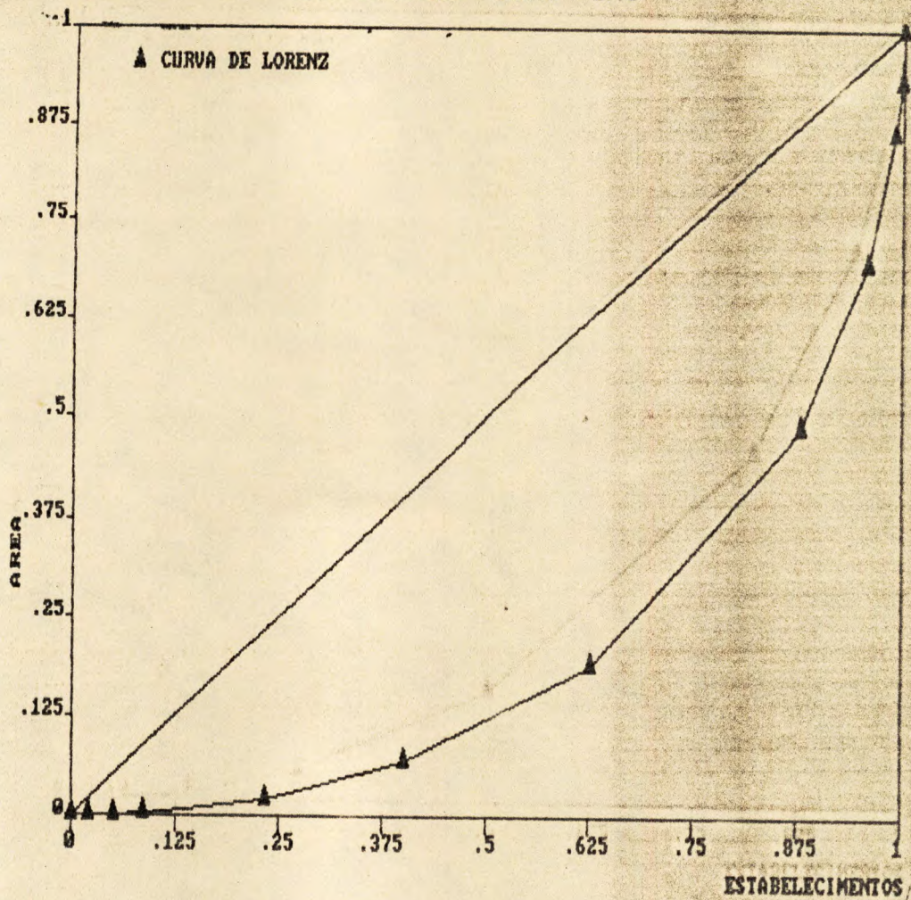
FIG.5: CURVA DE LORENZ PARA O MUNICÍPIO DE GURUPI (1970).
