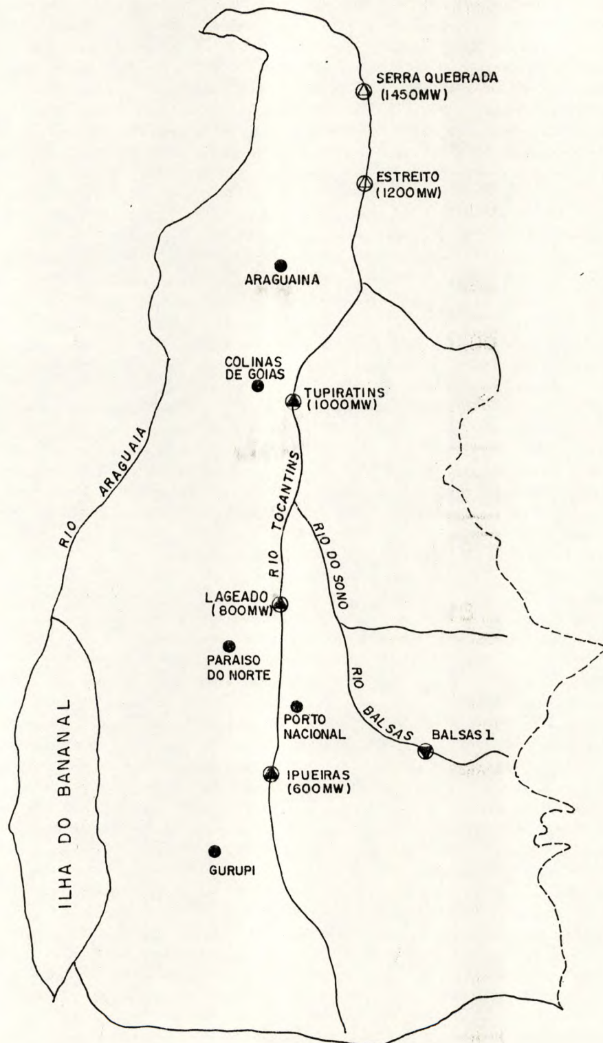
FIGURA 5.2.5-1 APROVEITAMENTOS INVENTARIADOS MÉDIO TOCANTINS
