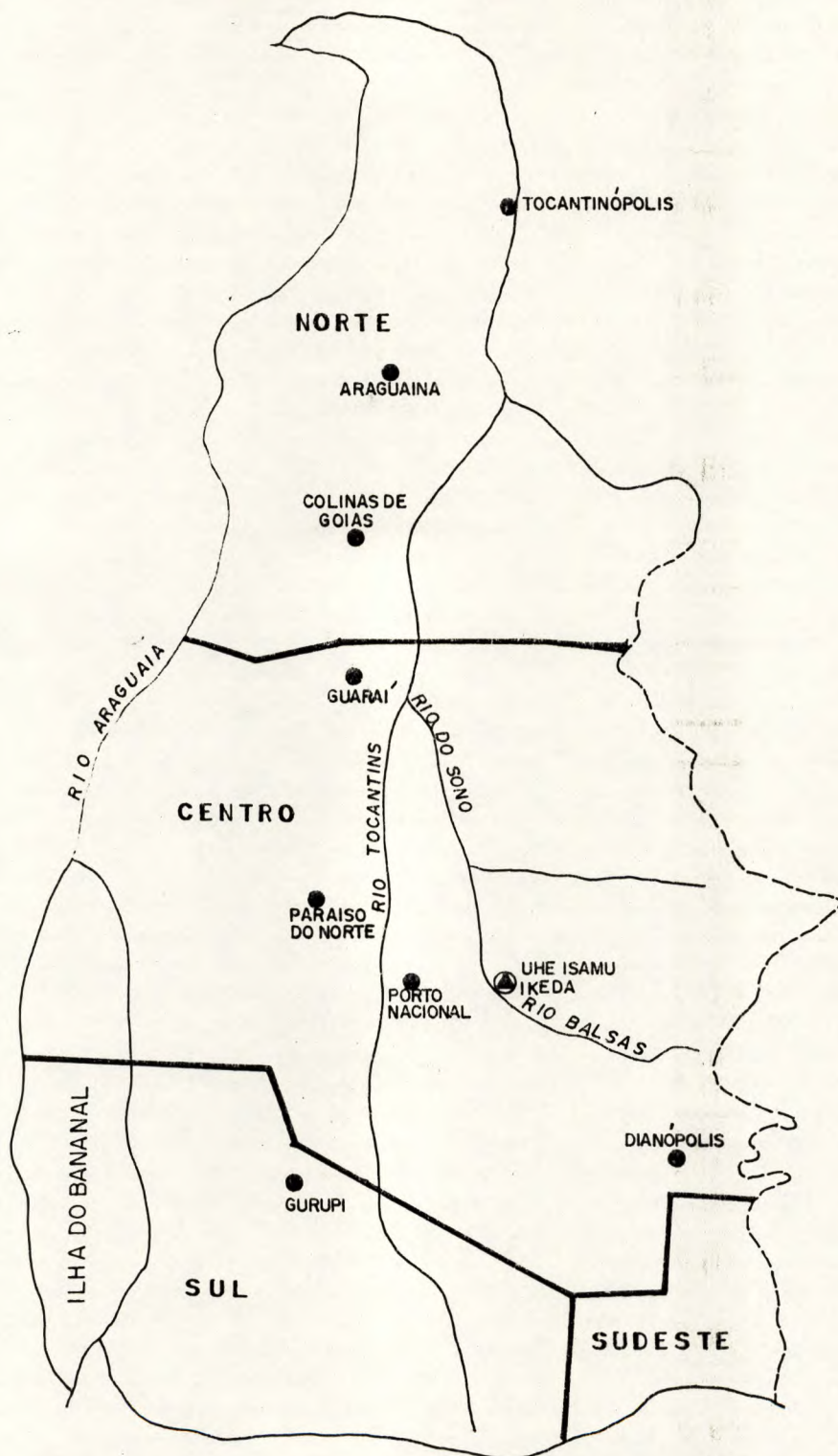
FIGURA 5.2.3-1 ESTADO DE TOCANTINS - ZONAS ELÉTRICAS
