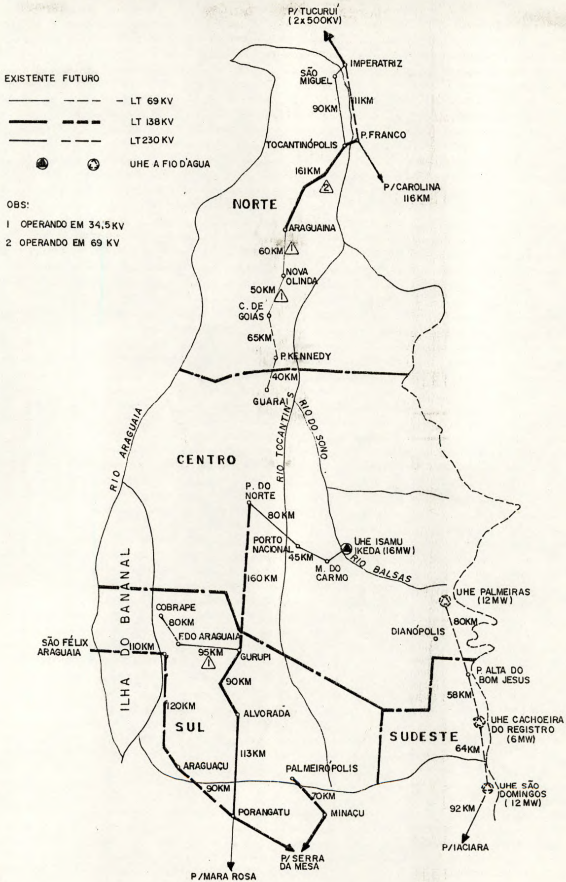
FIGURA 5.2.4-1 ESTADO DE TOCANTINS-MAPA ELETROGEOGRÁFICO PRINCIPAIS TRONCOS
