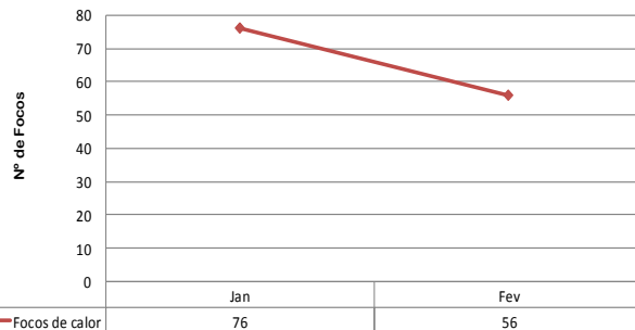
Focos de Calor - Estado de Tocantins (01/01/2021 a 27/02/2021)
