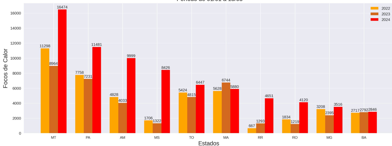
Comparativo dos Focos de Calor - Brasil Ranking PARCIAL dos estados (2022 a 2024) Período de 01/01 a 18/08
