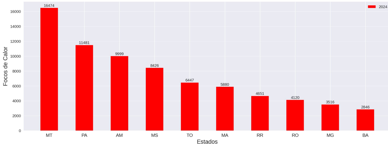
Focos de Calor - Brasil Ranking PARCIAL dos estados Período de 01/01 a 18/08
