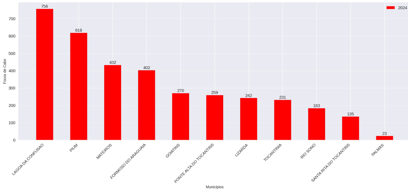
Focos de Calor - Tocantins Ranking dos municípios Período de 01/01 a 18/08
