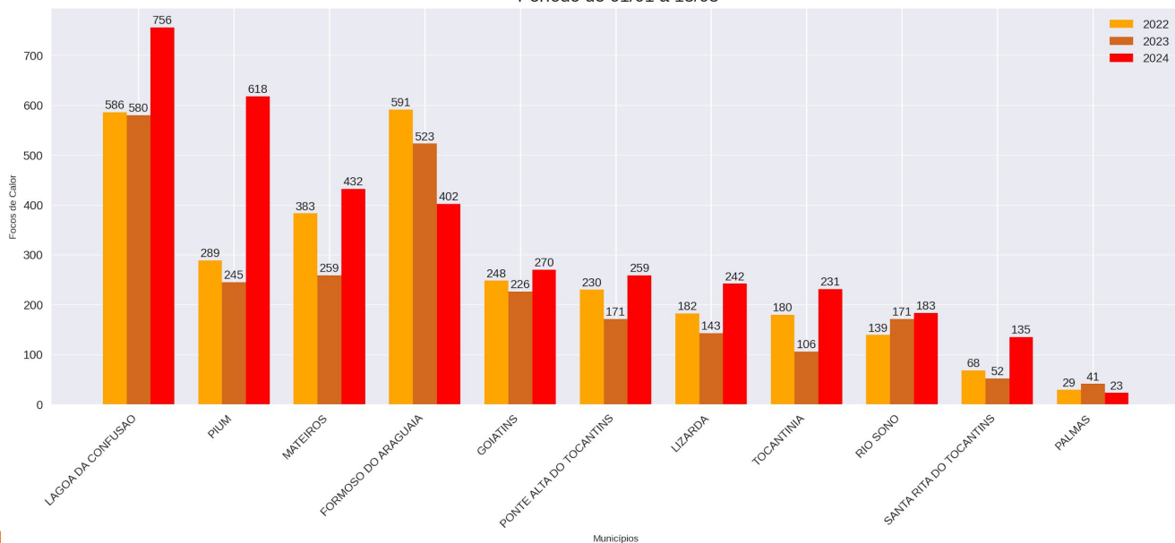
Comparativo dos Focos de Calor Ranking PARCIAL dos Municípios (2022 a 2024) Período de 01/01 a 18/08
