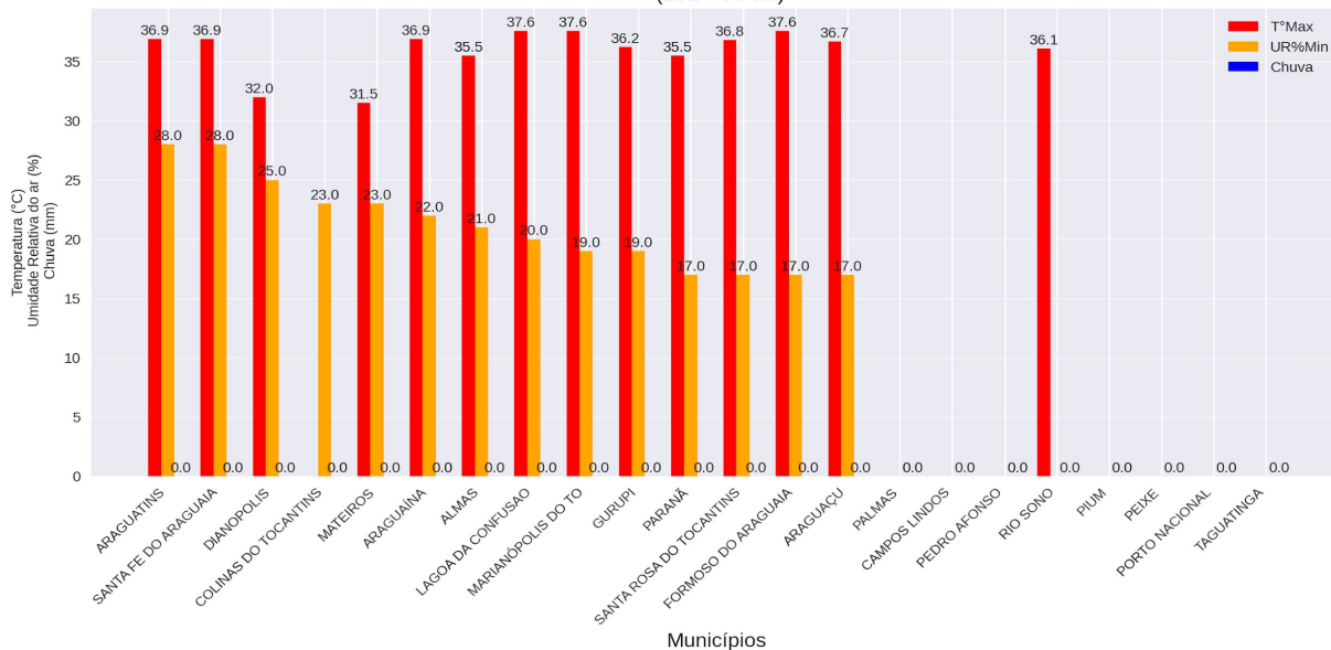
Registro Meteorológico (INMET) - Tocantins (2024-08-18)
