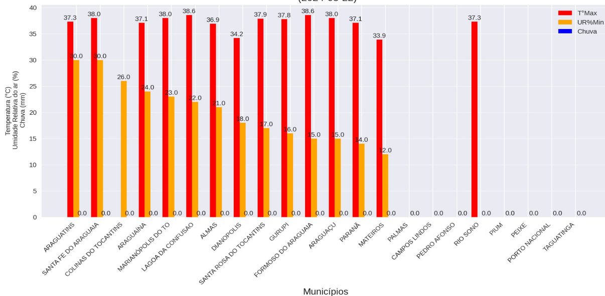
Registro Meteorológico (INMET) - Tocantins (2024-08-22)
