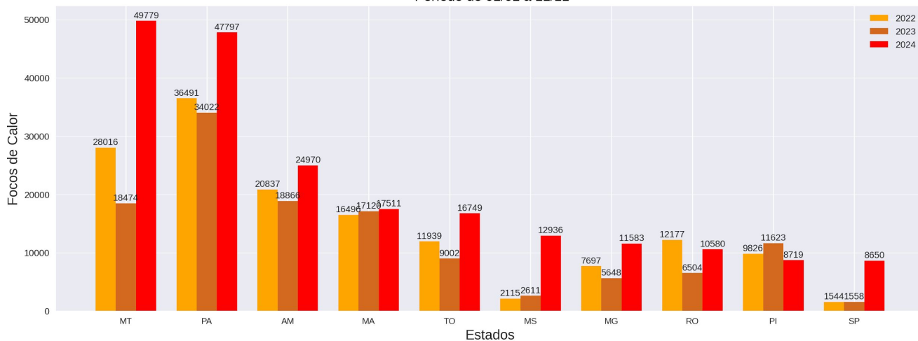
Comparativo dos Focos de Calor - Brasil Ranking PARCIAL dos estados (2022 a 2024) Período de 01/01 a 11/11
