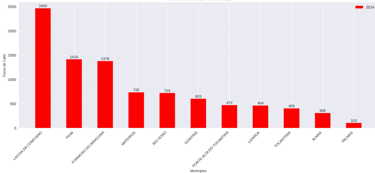
Focos de Calor - Tocantins Ranking dos municípios Período de 01/01 a 20/11
