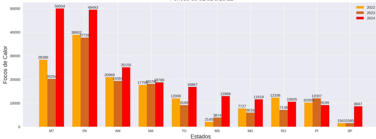
Comparativo dos Focos de Calor - Brasil Ranking PARCIAL dos estados (2022 a 2024) Período de 01/01 a 20/11
