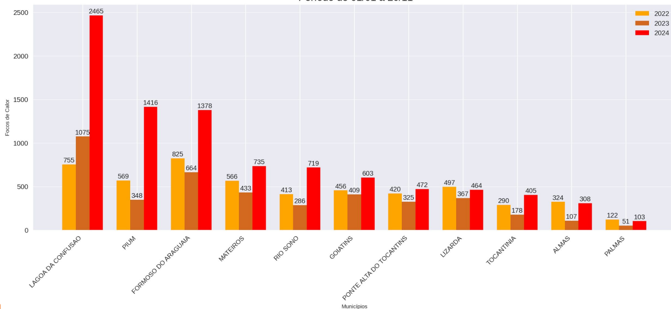
Comparativo dos Focos de Calor Ranking PARCIAL dos Municípios (2022 a 2024) Período de 01/01 a 20/11
