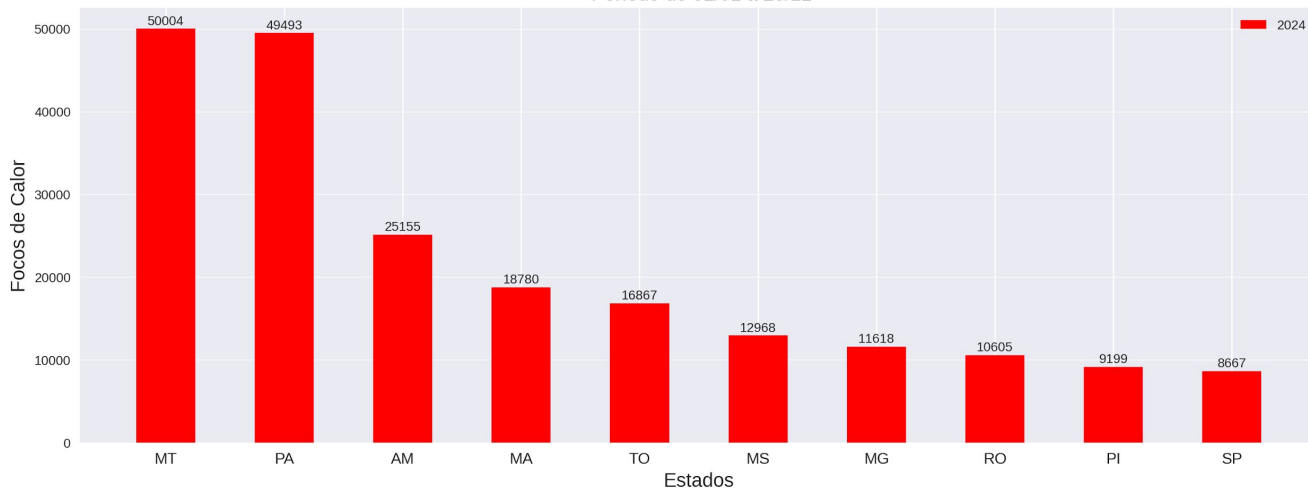
Focos de Calor - Brasil Ranking PARCIAL dos estados Período de 01/01 a 20/11
